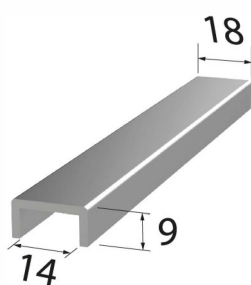
HR6 Pour verre 6+6 Main-Courante
