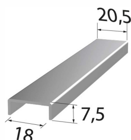
HR8 Pour verre 8+8 Main-Courante
